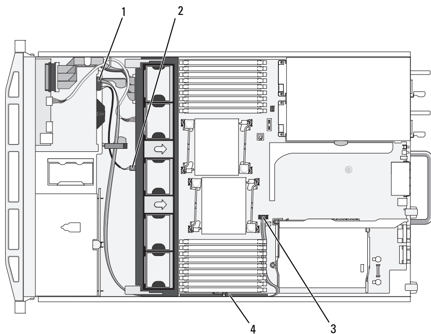
图 3-16. 布置光盘驱动器电缆 (3.5 英寸硬盘驱动器机箱)
