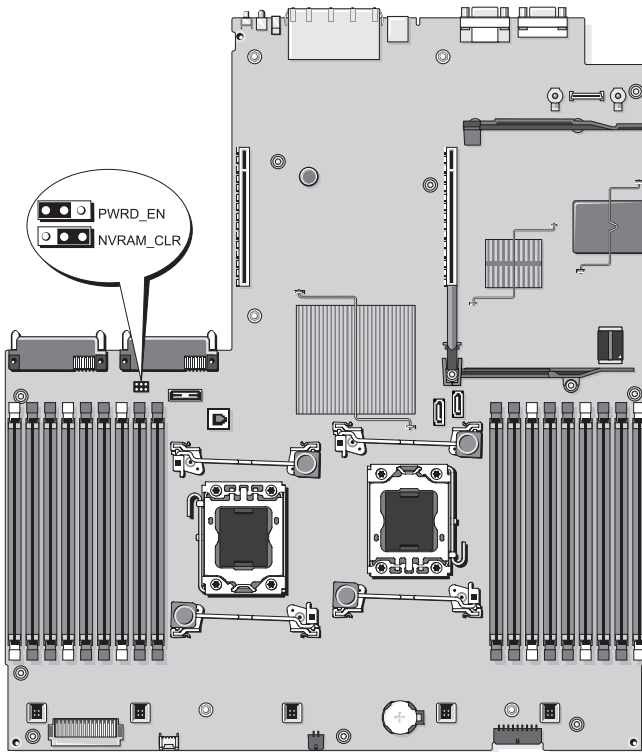
图 6-1. 系统板跳线
