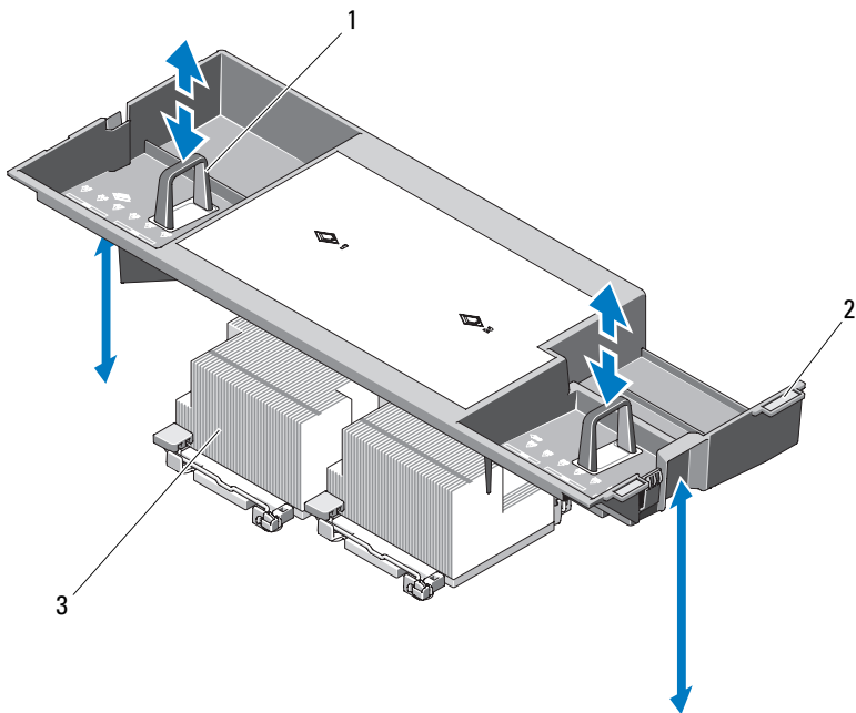
图 3-12. 卸下和安装冷却通风罩
