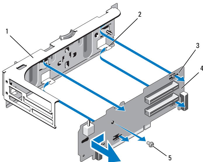
图 3-29. 卸下并安装提升板 2
