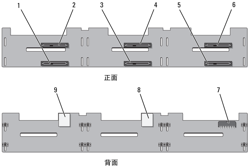
图 6-3. 3.5 英寸硬盘驱动器的 SAS 背板 (6 个插槽)
