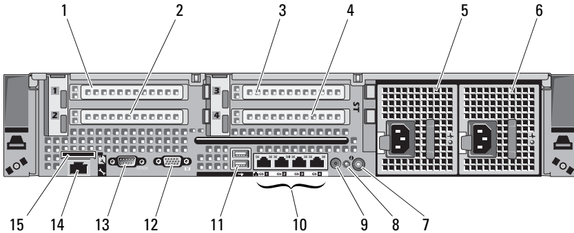
图 1-4. 背面板部件
