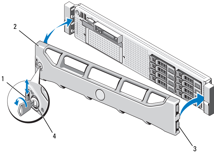
图 3-2. 卸下前挡板
