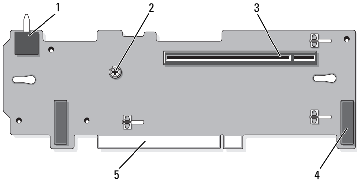
图 6-6. 可选 PCIe x16 扩充卡提升板 2 组件
