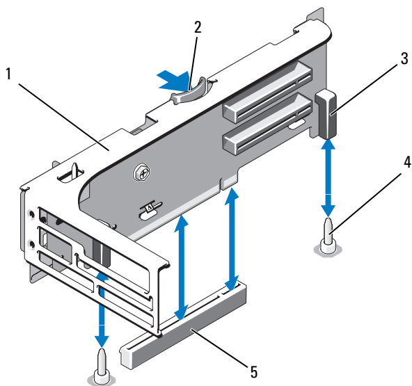
图 3-28. 卸下和安装扩充卡提升板 2
