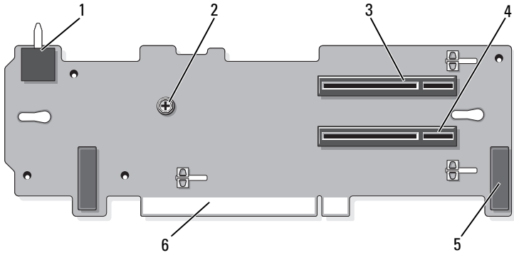
图 6-5. 标准 PCIe 扩充卡提升板 2 组件
