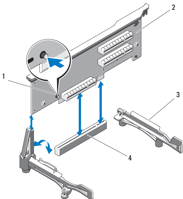
图 3-27. 卸下和安装扩充卡提升板 1
