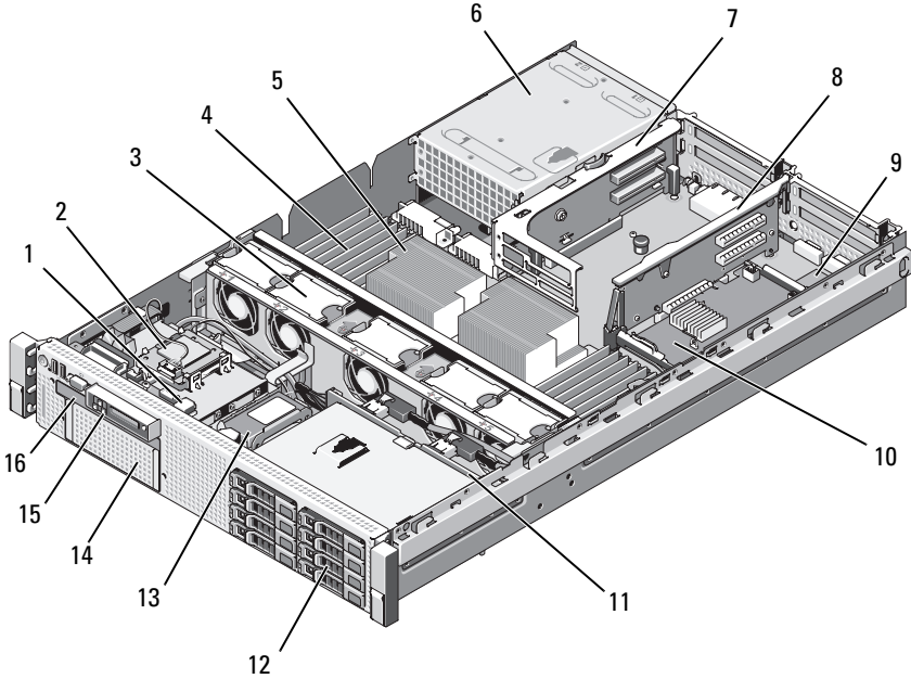
图 3-1. 系统内 (3.5 英寸硬盘驱动器机箱)
