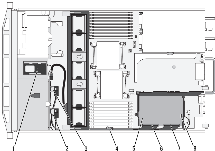
图 3-21. 存储控制器卡布线 (3.5 英寸硬盘驱动器机箱)
